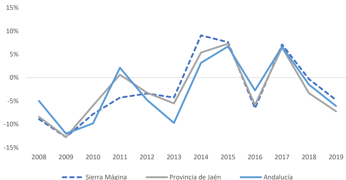
Gráfico 115. Emisiones de gases de efecto invernadero en t CO 2 equivalente – Variación interanual (%)
