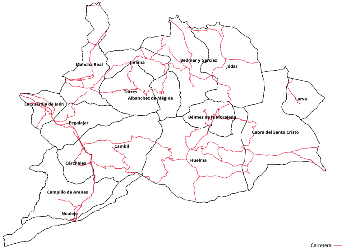
Mapa 29. Red de carreteras
