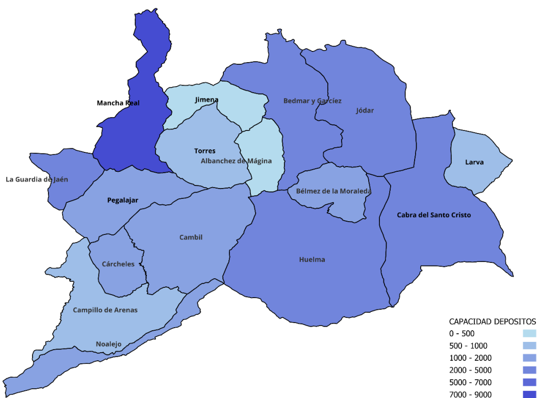
Mapa 24. Capacidad de los depósitos de agua (metros cúbicos)
